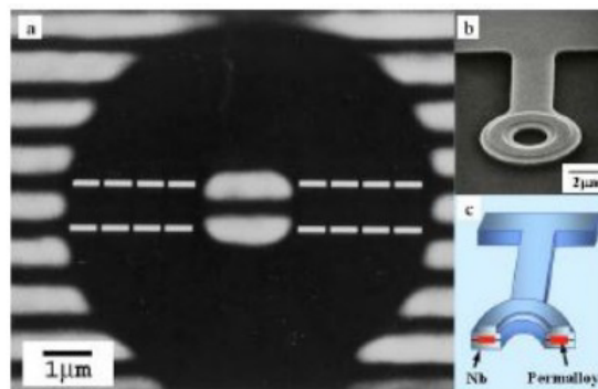
Figura 3.5: a) Franjas de interferência do feixe de elétrons, diferença de fase gerado pelo vetor potencial sobre os elétrons. b e c) Imagem do pequeno toroide [52]
