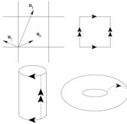
Figura 2.4: Espaço do parâmetro de ordem dos deslocamentos atômicos em uma rede quadrada.
