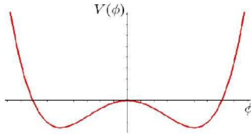
Figura 2.2: Potencial escalar V(\phi) , quando \mu^2 < 0 .
