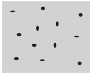
Figura 3.5: Representação esquemática de defeitos tipo monopolos.
