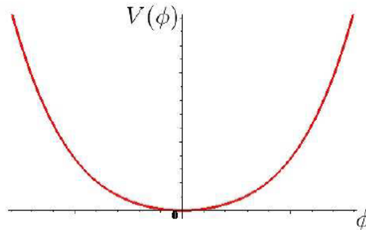
Figura 2.1: Potencial escalar V(\phi) , quando \mu^2 > 0 .
