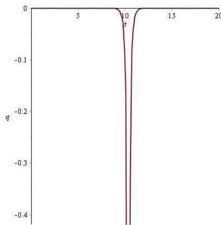
Figura 4.13: Evolução do parâmetro de desaceleração em função do tempo. Para o universo dominado pela poeira percebe-se fase acelerada do universo, assumimos A = 1 e t_0 = 10 .
