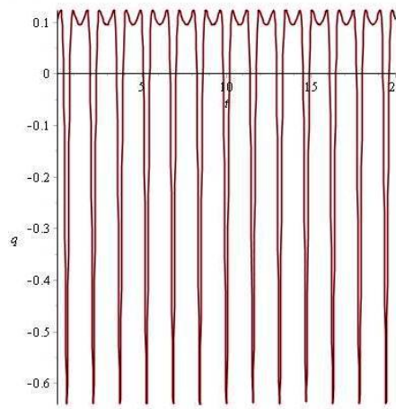
Figura 4.17: Evolução do parâmetro de desaceleração em função do tempo. Para o universo dominado pela radiação percebe-se curtos intervalos de aceleração e desaceleração do universo, assumimos A = 1 e t_0 = 10 .
